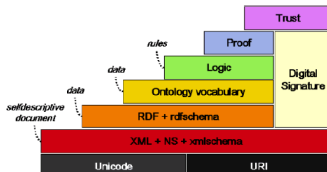
FIG. 1 – Les couches du Web sémantique
